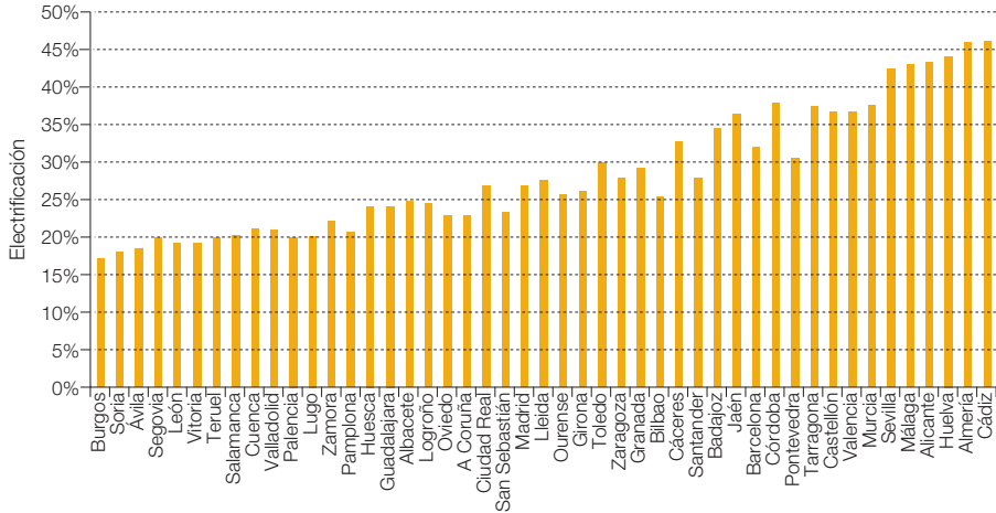
Figura 259. Electrificación en viviendas bloque parque actual.
