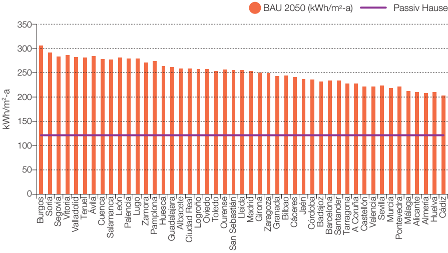
Figura 261. Consumo medio de energía primaria total en viviendas unifamiliar parque BAU 2050.
