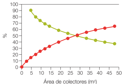
Solar para ACS &amp; calefacción
